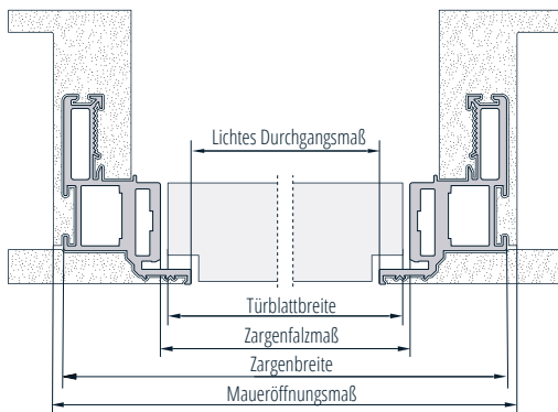
Variante DRÜCKEN
